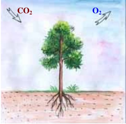
ព្រៃឈើស្រូបយកឧស្ម័ន CO 2 ពីបរិយាកាស
